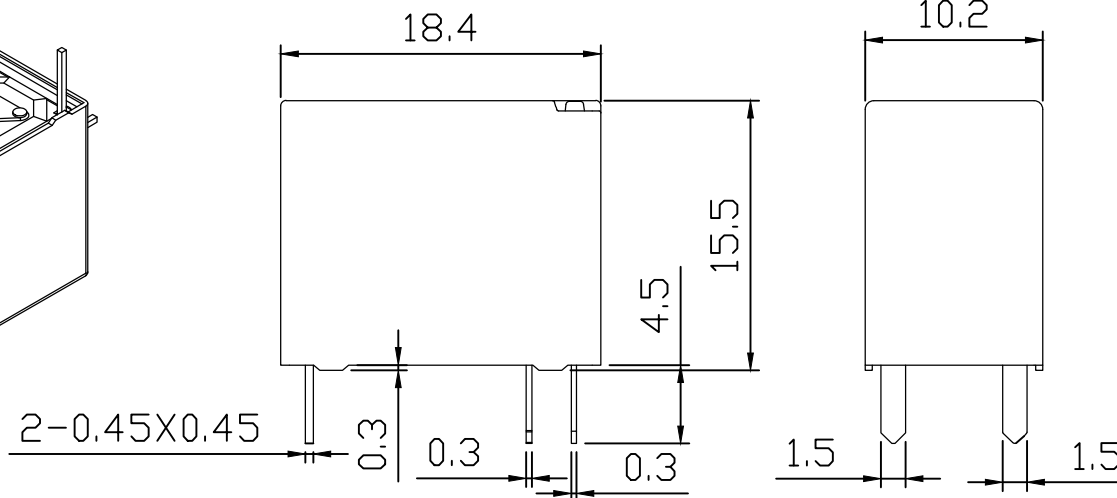
主视图
